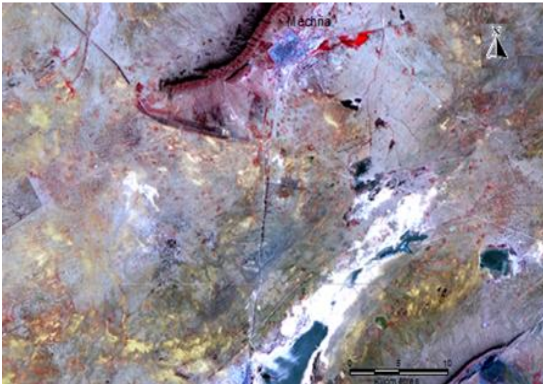
Figure n°11: la composition colorée
