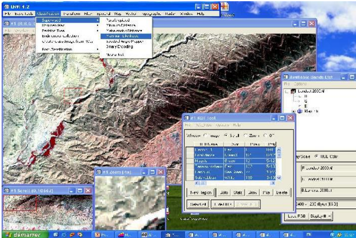
Figure n°12: Technique de la classification et de la composition colorée
